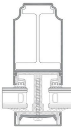
VT+ külső szaruelem keresztmetszet
